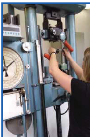
Meranie nosnosti oceľového drôtu Measurement of axial load the steel wire
